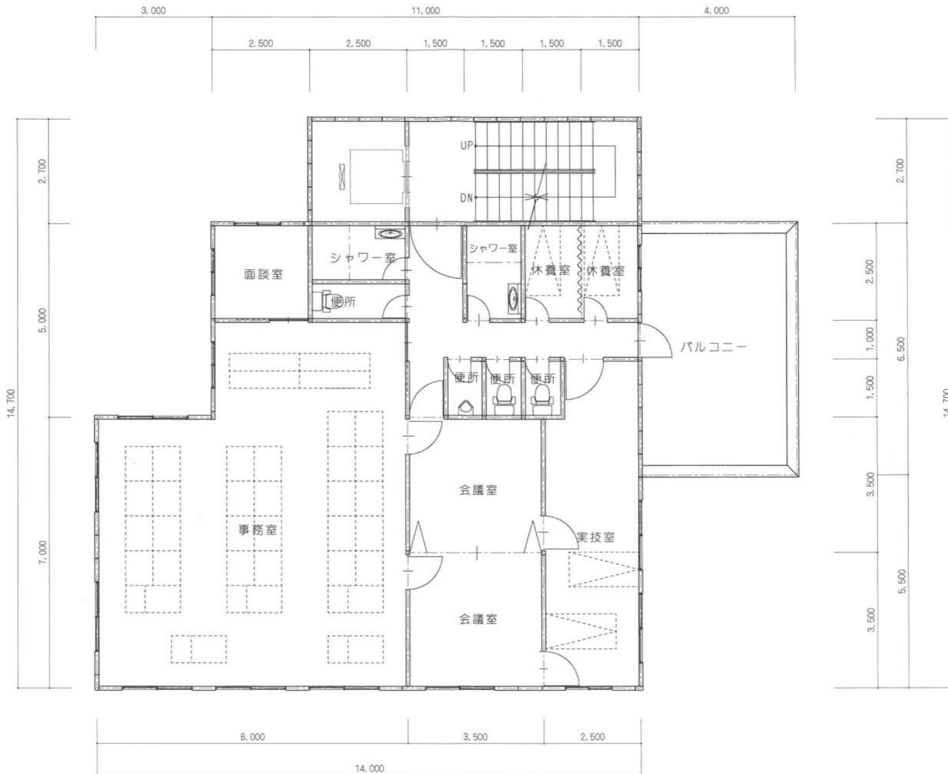
2階平面図
